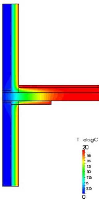
Modélisation d'un pont thermique de plancher intermédiaire
